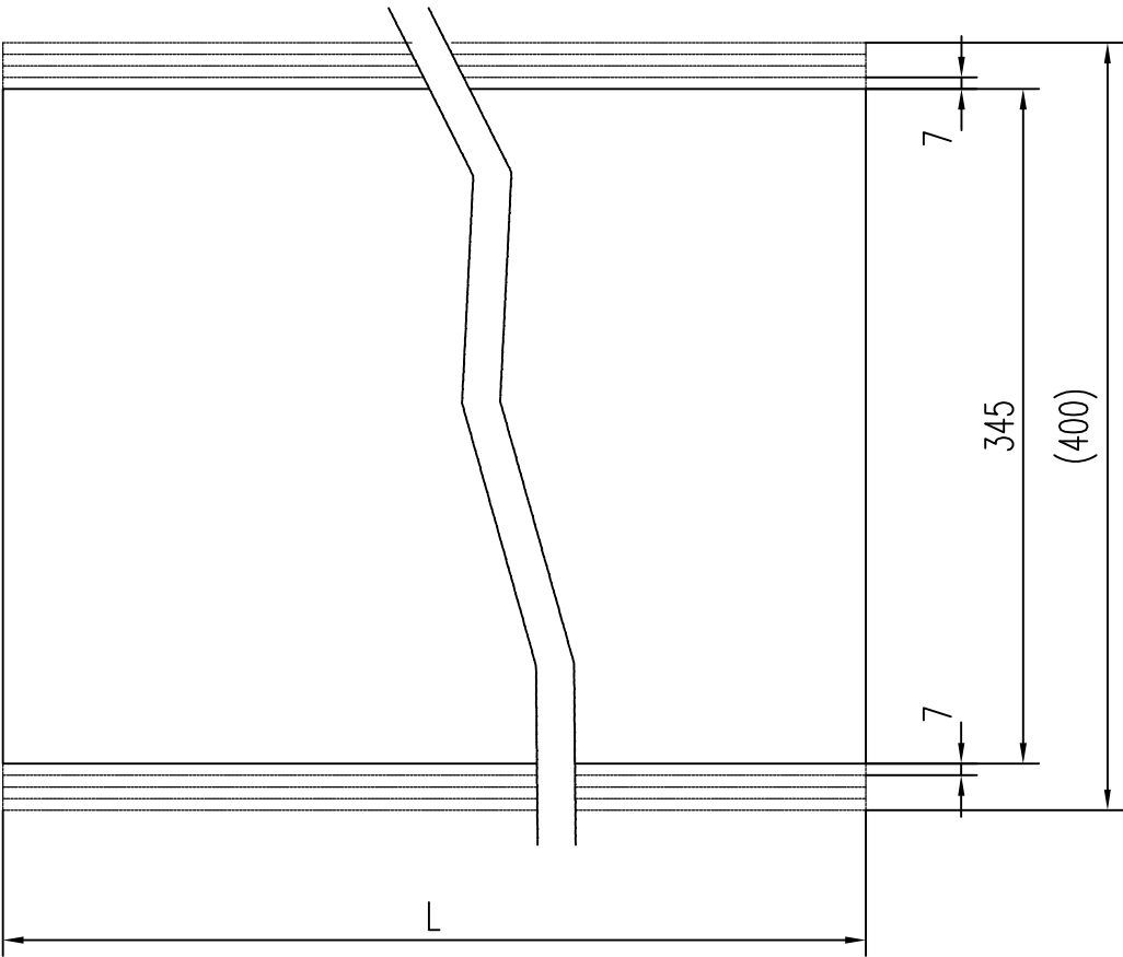
层间绝缘展开宽参考尺寸
